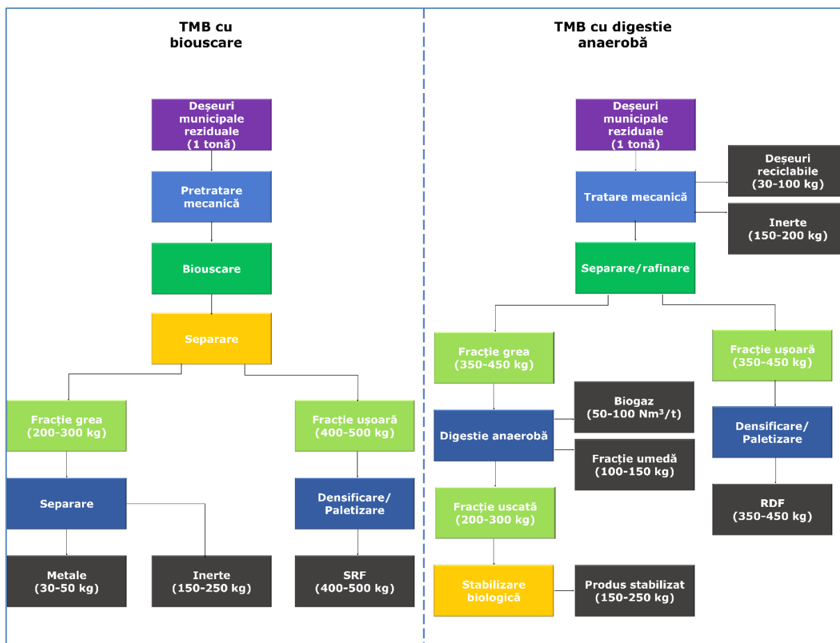
Figura 7-1: Fluxul tehnologic al instalațiilor TMB cu bioscare și digestie anaerobă 61
