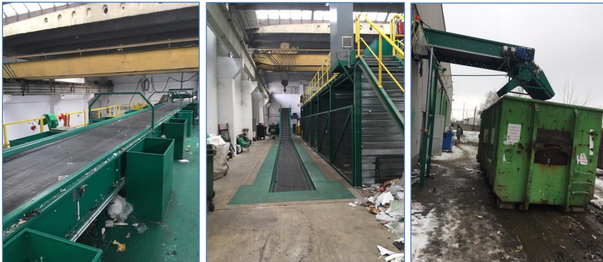
Figura 4-14: Stație de sortare S.C. RER Ecologic Service REBU S.A.
