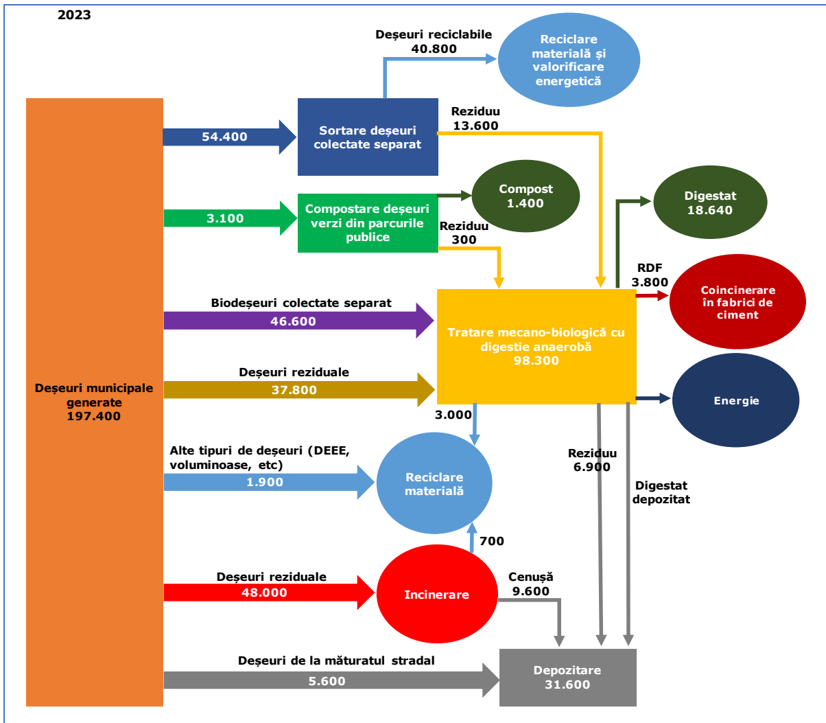
Figura 7-16: Schema fluxului de deșeurii în alternativa selectată (Alternativa 2), 2023
