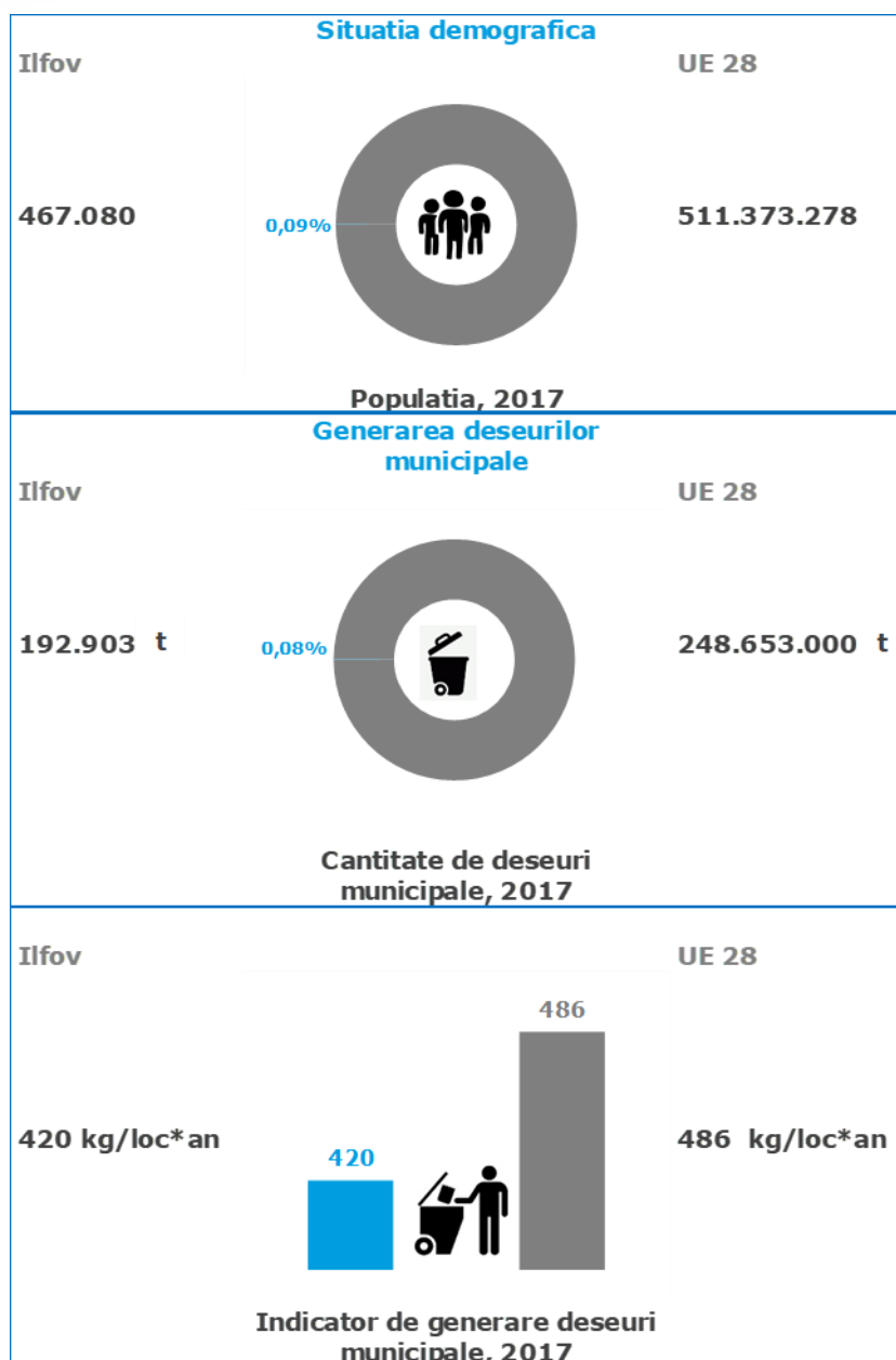
Figura 4-5: Generarea deșeurilor municipale 2017, Ilfov versus UE 28
