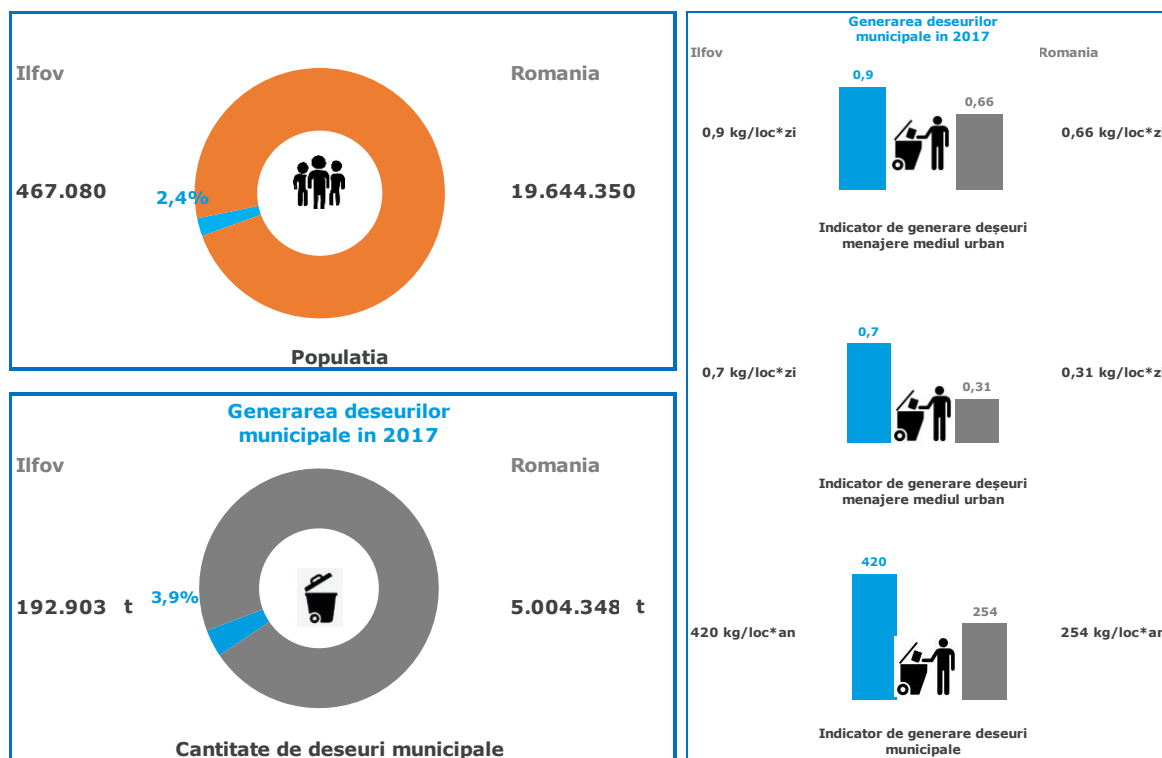
Figura 4-4: Generarea deșeurilor municipale 2017, Ilfov versus România
